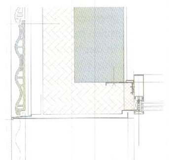
Fassadenschnitt
